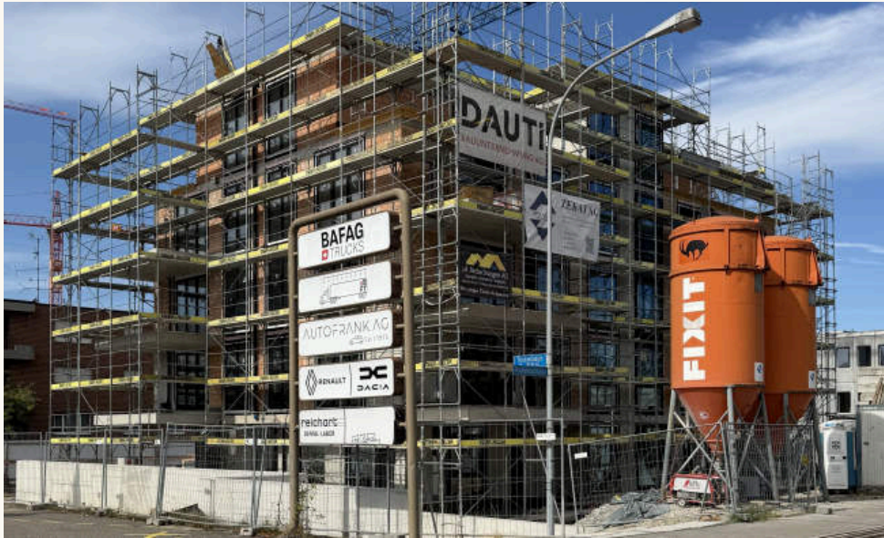
1 Baustelle an der Trockenloostrasse, September 2026: der Rohbau in Backstein und Stahlbeton im Gerüst, die Fensteröffnungen gesetzt; davor die Kranbahn und die Silos des Baumeisters. Foto: Ivanov + Partners
