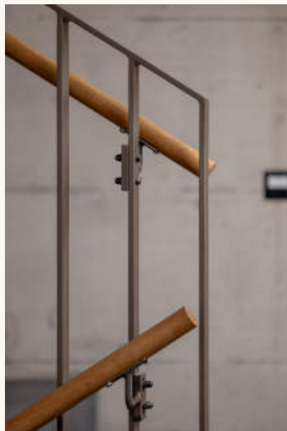
4 Balkonzone im Abendlicht: Betonbänder, Stahlstützen und Staketengeländer vor den raumhohen Verglasungen; Senkrechtmarkisen als Sonnenschutz. 5 Treppenhaus: Geländer aus Flachstahl mit Handlauf in Eiche vor Sichtbeton, die Verbindungen sichtbar verschraubt. Foto: foter.sk
